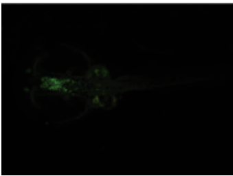
Fig. 1: Gène peu exprimé
