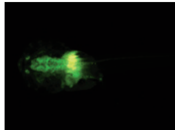
Fig. 2: Gène fortement exprimé
