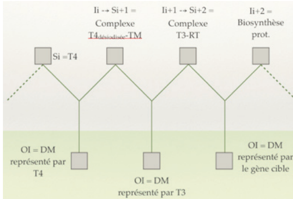
Fig. 3: Processus sémiosique de la morphogenèse liée à l'hormone T4 de Xenopus Laevis
